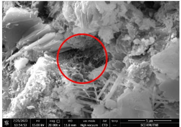
รูปที่ 3 และ รูปที่ 4 ภาพถ่าย SEM ที่กำลังขยาย 20,000 เท่า ที่ตำแหน่งแตกต่างกัน
